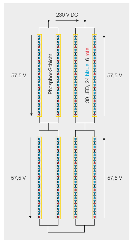
Bild 2 Vereinfachtes Schaltschema einer Filament-Lampe: Die insgesamt acht Leuchtfäden sind paarweise in Serie geschaltet. Die Betriebsspannung beträgt 57,5 V Gleichstrom, was einen Gleichrichter im Schraubsockel bedingt. In dieser Konfiguration leuchten im Betrieb 240 LED.
