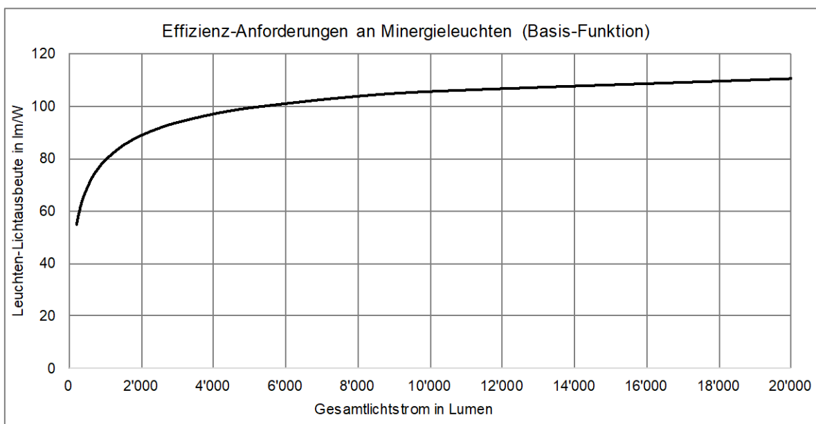
Bild: Effizienz-Anforderungen an Minergie-Leuchten (Leuchtyp 1, 4000 K, CRI = 80)
